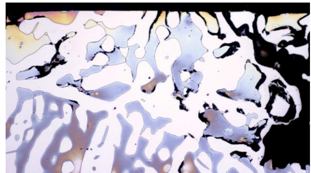
Selektive Korrosion an einem Pumpengehäuse aus Duplexstahl in einer Rauchgasreinigungsanlage (Lichtmikroskopie)
